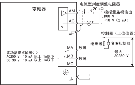
图 3.19 接点输出
