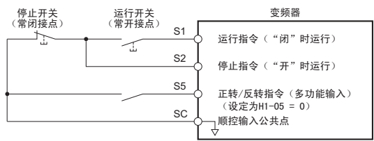
图 3.2 3 线制顺控
