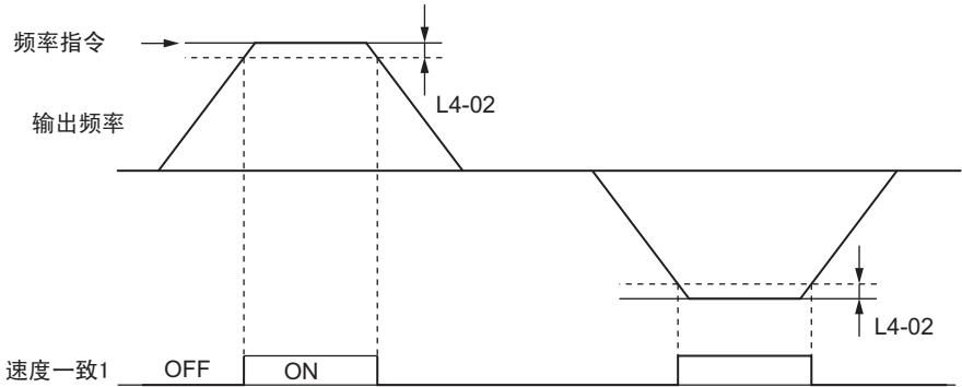
图 5.19 速度一致 1 的时序图
