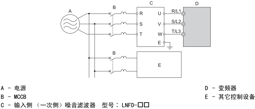
图 8.7 输入侧（一次侧）噪音滤波器的连接示例（三相 200 V/400 V）
