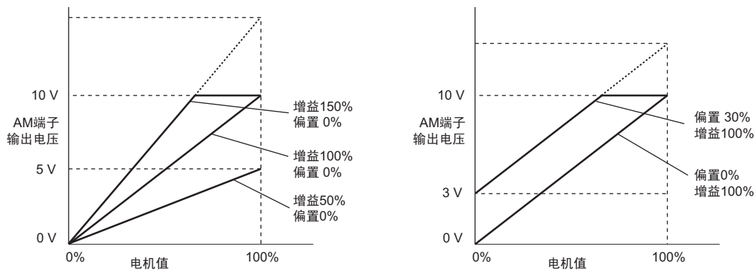
图 5.29 模拟量输出的增益 / 偏置设定
