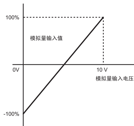
图 5.24 无 0 极限的模拟量输入（偏置设定 -100%）
