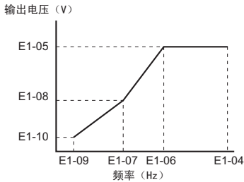
图 5.11 V/f 曲线图
