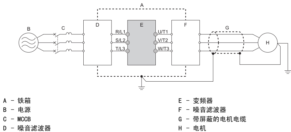
图 8.10 无线电干扰防止对策
