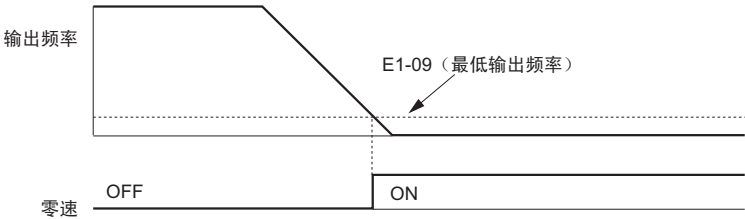
图 5.18 零速的时序图
