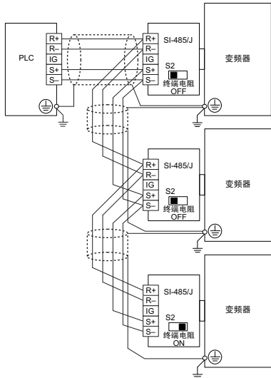
图 C. 4 使用 RS-422 通信时的接线
