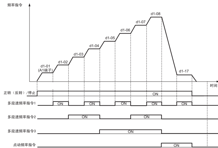
图 5.7 多段速指令 / 点动频率选择的时序图
