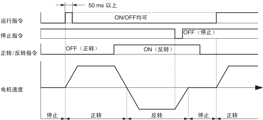
图 5.13 3 线制顺控的时序图
