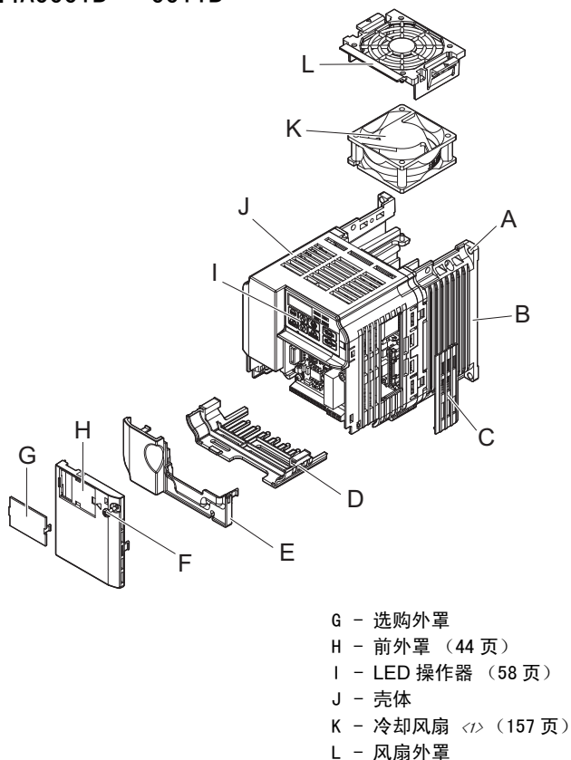
图 1.3 柜内安装型变频器各部分的名称 CIMR-J□2A00012B
