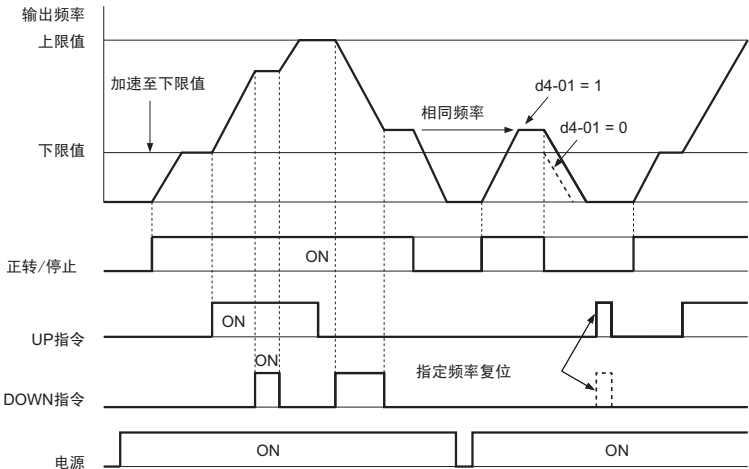
图 5.15 UP/DOWN 指令的时序图
