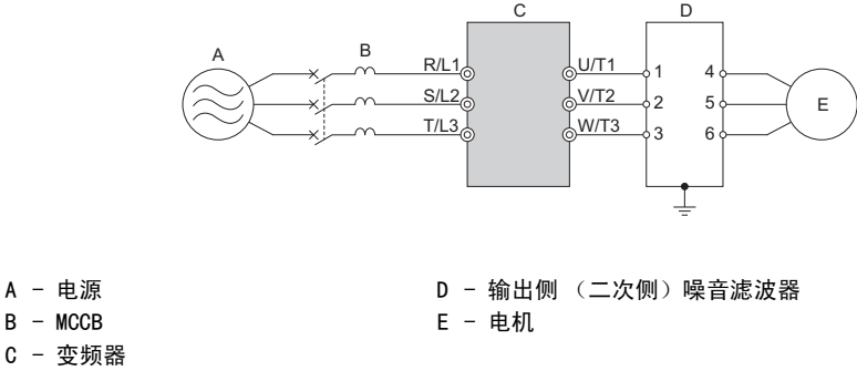
图 8.8 输出侧（二次侧）噪音滤波器的连接示例
