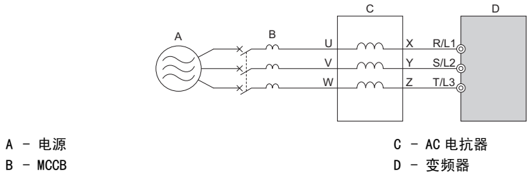
图 8.4 AC 电抗器的连接示例
