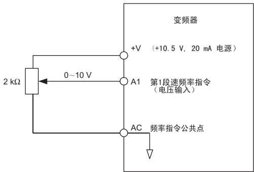
图 5.1 第 1 段速频率指令的电压输入
