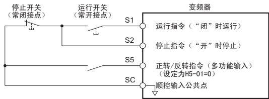
图 5.12 3 线制顺控的接线示例
