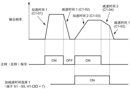
图 5.3 加减速时间的时序图
