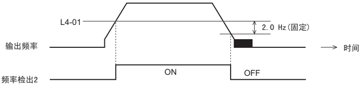
图 5.34 频率检出 2
