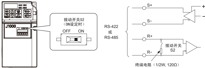
图 C. 5 MEMOBUS 通信端子与拨动开关 S2
