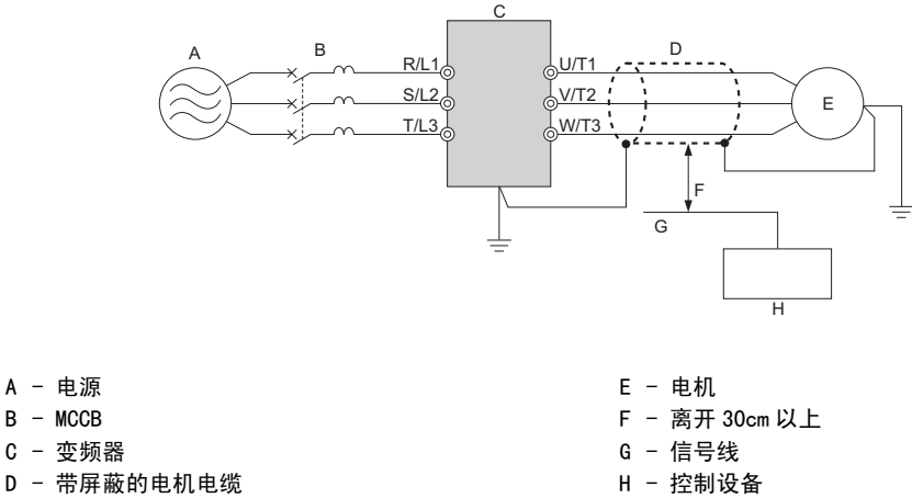
图 8.9 感应干扰防止对策
