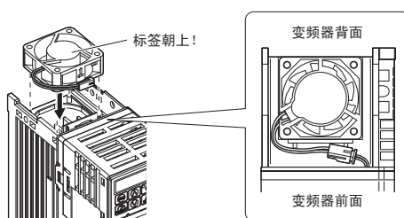
图 7.2 冷却风扇的安装方向
