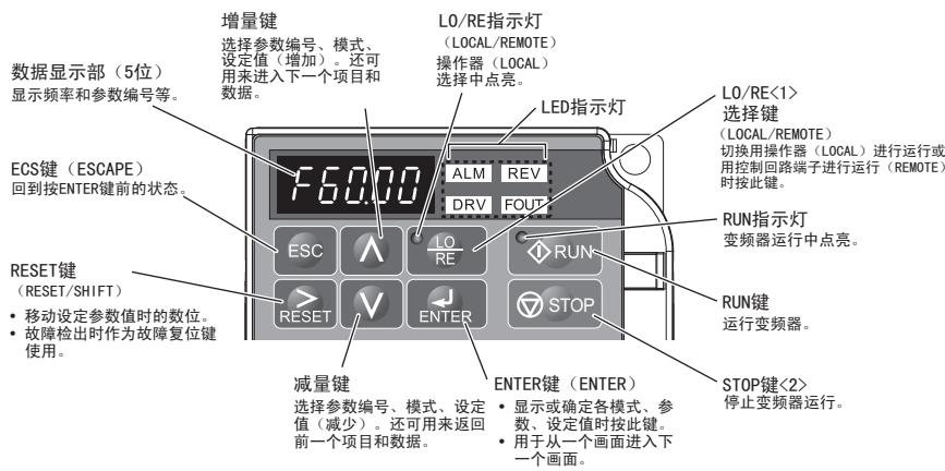
图 4.1 LED 操作器各部分的名称与功能
