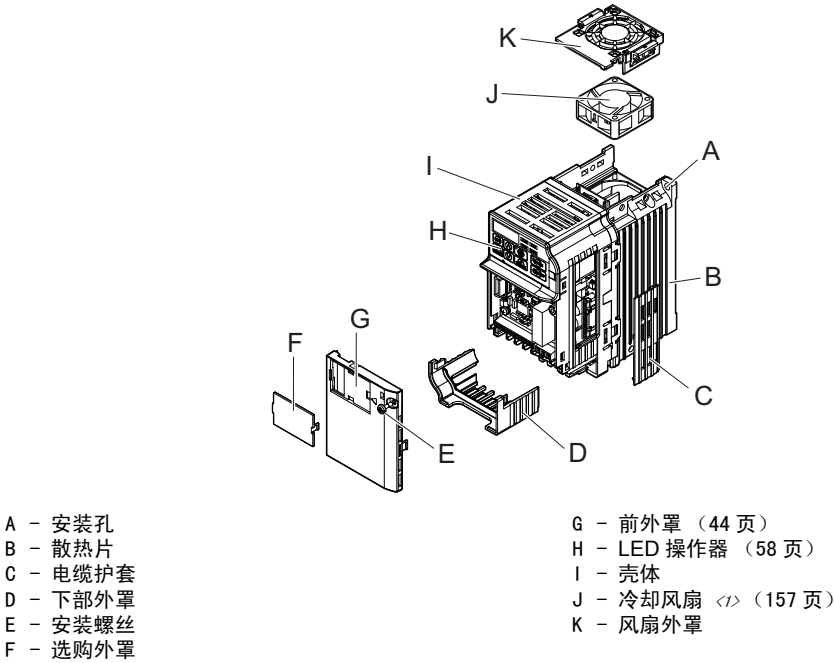
图 1.2 柜内安装型变频器各部分的名称 C1MR-J□2A0006B
