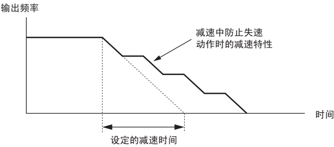
图 5.33 减速中防止失速的动作示例
