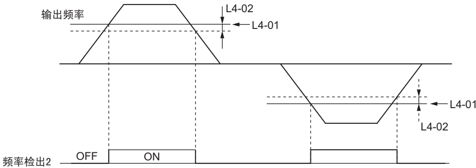
图 5.21 频率（FOUT）检出 2 的时序图
