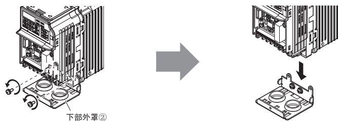
图 8.13 下部外罩的拆卸方法
