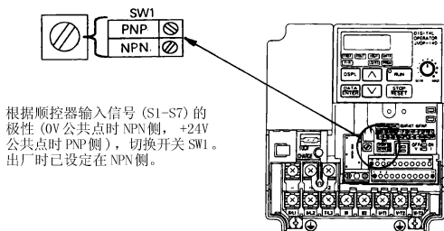
NPN 晶体管顺控器的接线图 (0V 公共点)
